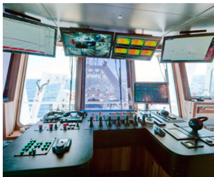
■ Stjórnþúlt fyrir vindukerfið.
